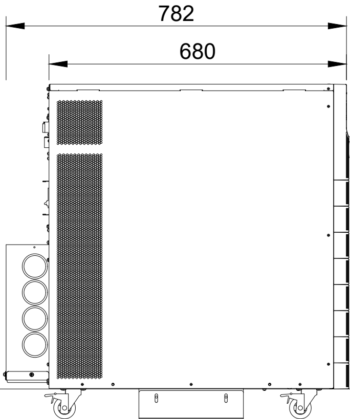
SIDE(L)
